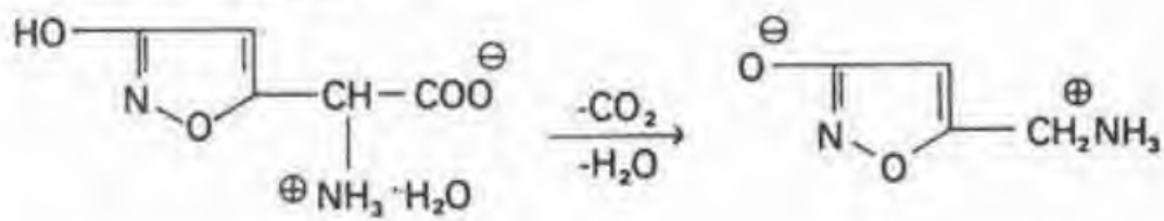
MUSCIMOLE
